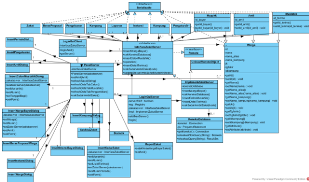
Gambar 5. Class Diagram Aplikasi zakat
