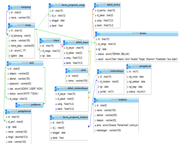
Gambar 9. Relasi Antar Tabel Zakat
